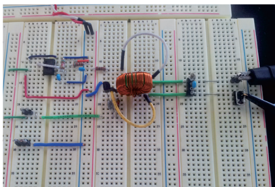
電子部品測定の様子① 電気計測を行うことで、電子部品の特性を学びます。
