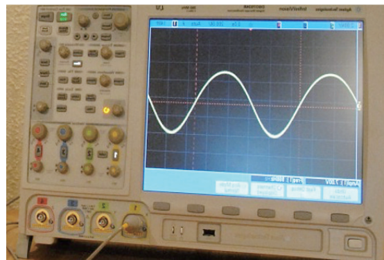
電子部品測定の様子② 実測により、計測器の使い方を学びます。
